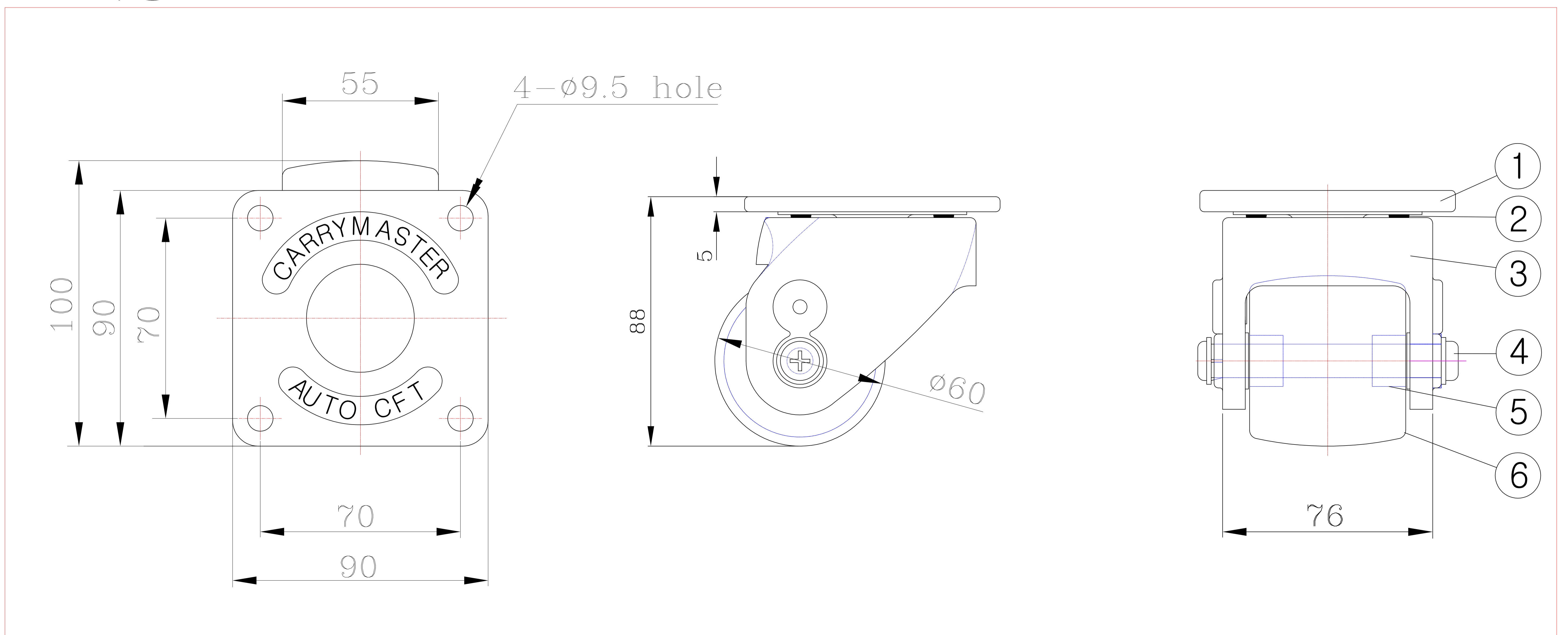
ACM-600FPU TYPE
